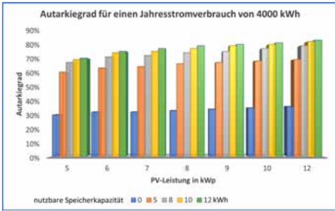
Bild 2: Simulation des Autarkiegrads für einen angenommenen Jahresstromverbrauch von 4000 kWh und einem spezifischen Jahresertrag von 1000 kWh/kWp in Abhängigkeit der installierten PV-Leistung und der nutzbaren Speicherkapazität.
